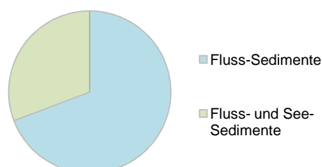
Abbildung 2: Herkunft der untersuchten natürlichen Sedimente (Antwort von 13 Kantonen).
